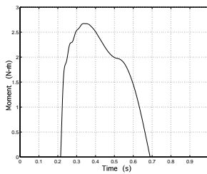
Fig. 9. Contact Torque.
