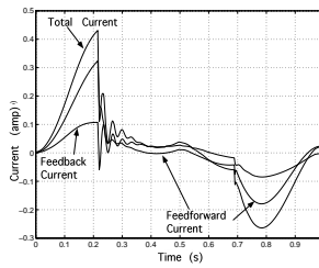
Fig. 10. Current Input.
